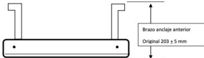
Estructura secundaria Toyota Etios, dimensiones, tolerancia +/- 5mm
