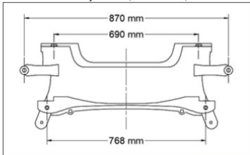
Estructura secundaria Toyota Etios, dimensiones, tolerancia +/- 5mm
